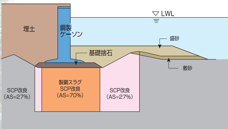
●サンドコンパクションパイル
