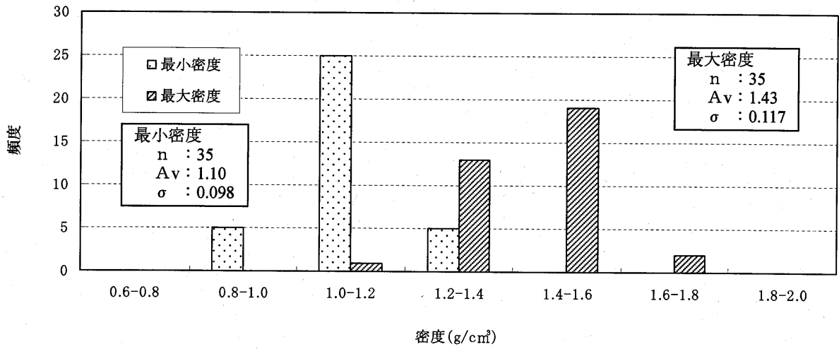
図 3.1.2 水砕スラグの最大・最小密度
