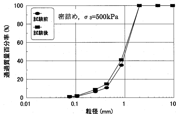
図 3.1.15 三軸圧縮試験前後の粒度の変化(拘束圧 500kPa) 14)
