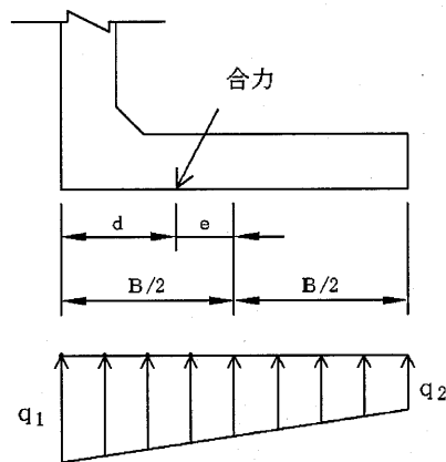
図 5.1.4 地盤反力
