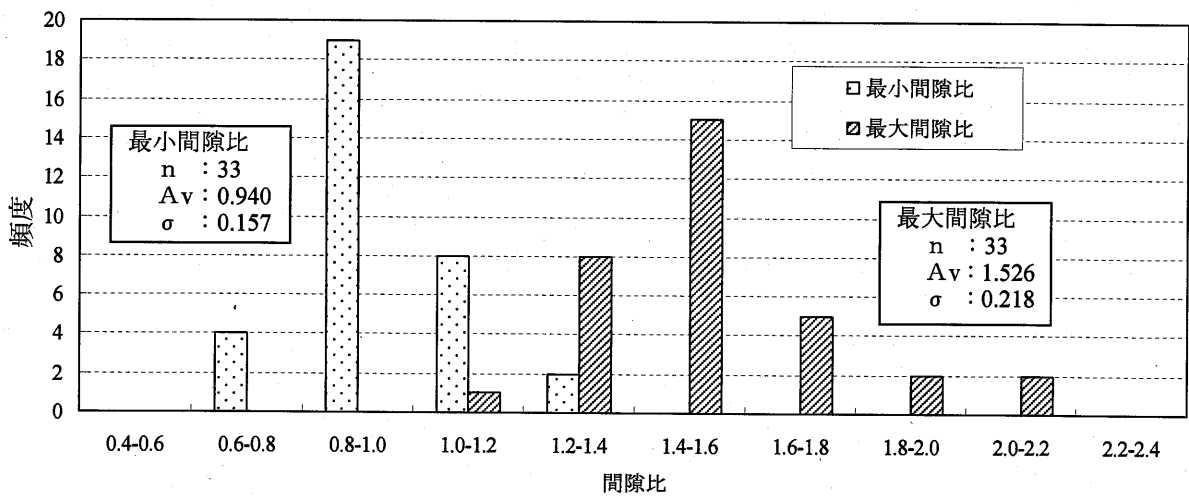
図 3.1.3 水砕スラグの最大・最小間隙比
